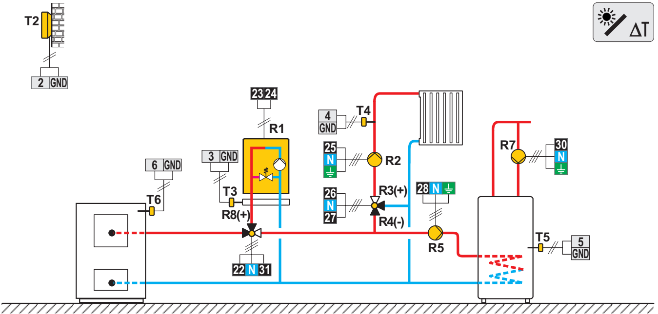
Scheme 408b (WDC20) - Chaudière à combustible solide, chaudière à gaz, circuit mélangeur, chauffe-eau sanitaire
