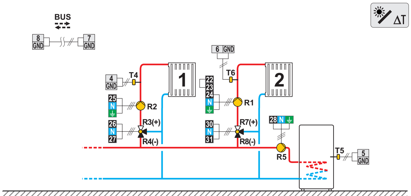
Schema 423h (WDC20) - Schéma d'extension, 2x circuit mélangeur, chauffe-eau sanitaire.
