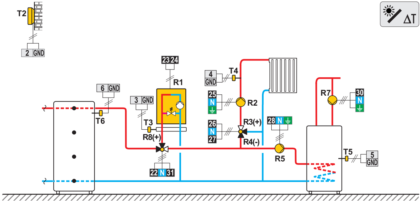
Scheme 409b (WDC20) - Ballon d'eau chaude, chaudière à gaz, circuit mélangeur, chauffe-eau sanitaire
