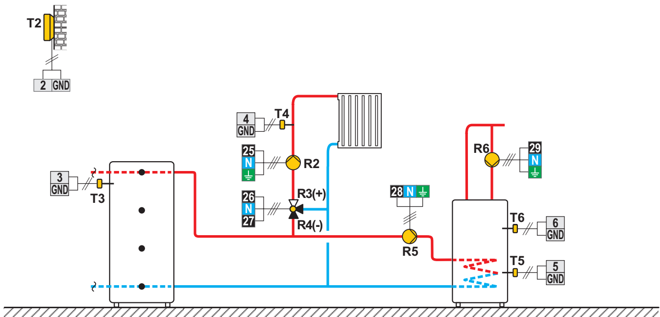
Scheme 401b (WDC10B, WDC10, WDC20) - Ballon d'eau chaude, circuit mélangeur, chauffe-eau sanitaire
