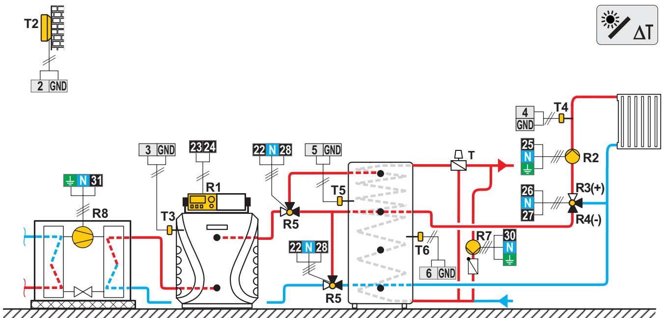
Scheme 422d (WDC20) - Pompe à chaleur, chaudière à fioul, ballon d'eau chaude avec chauffe-eau, sanitaire, circuit mélangeur
