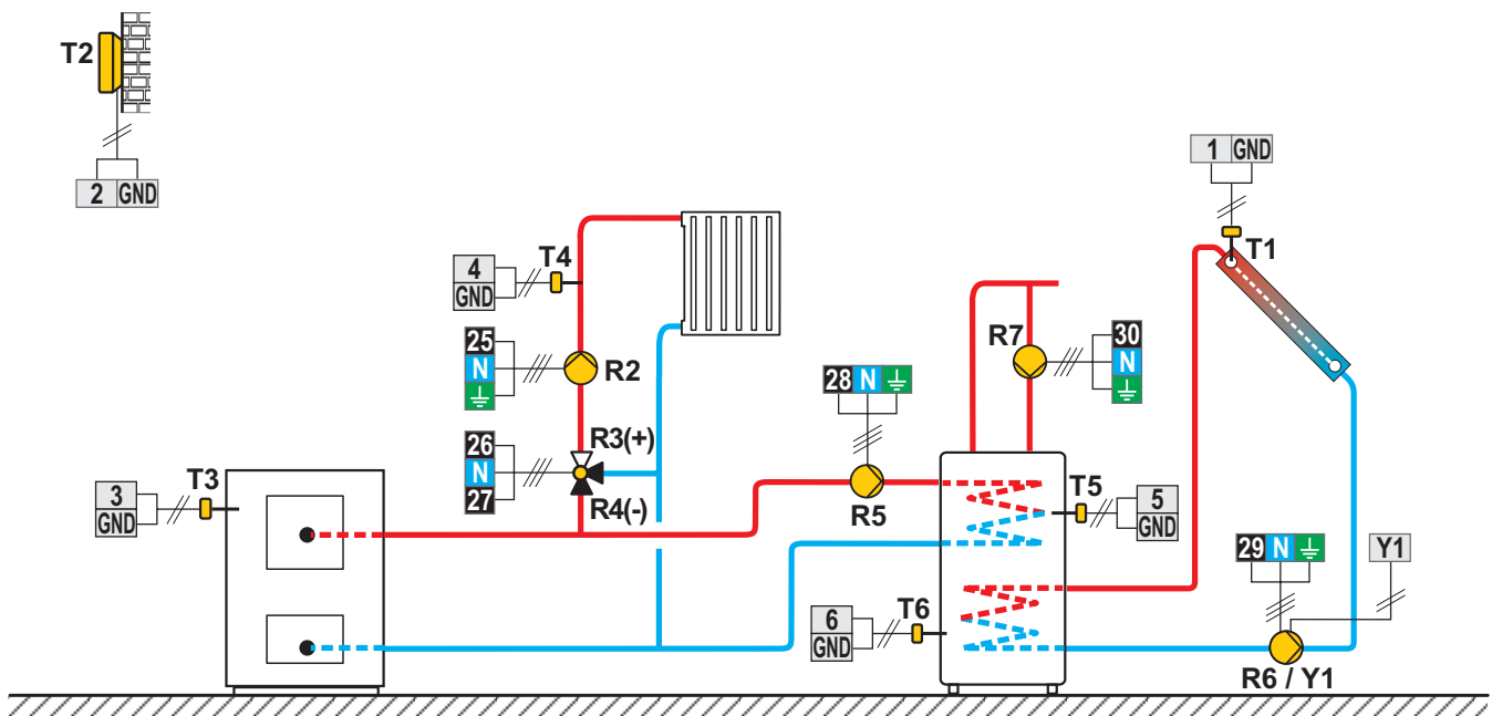
Scheme 404c (WDC10, WDC20) - Chaudière à combustible solide, circuit mélangeur, chauffe-eau sanitaire, capteurs solaires
