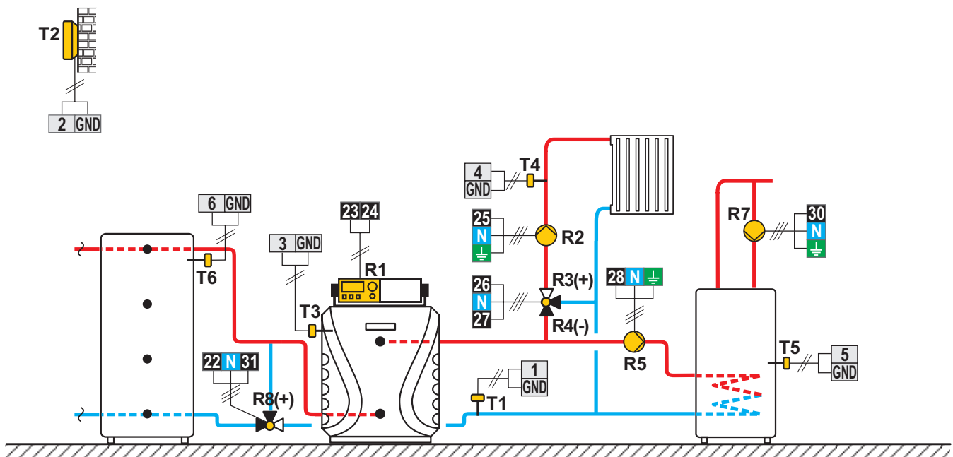
Scheme 410 (WDC20) - Ballon d'eau chaude, chaudière à fioul, circuit mélangeur, chauffe-eau sanitaire
