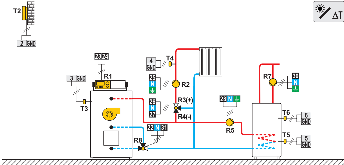
Scheme 418 (WDC20) - Chaudière combinée (combustible solide/fioul), circuit mélangeur, chauffe-eau sanitaire
