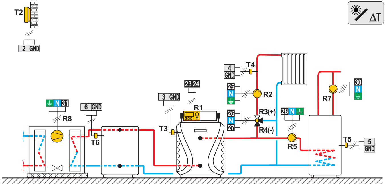
Scheme 422c (WDC20) - Pompe à chaleur, chaudière à fioul, ballon d'eau chaude, circuit mélangeur chauffe-eau sanitaire
