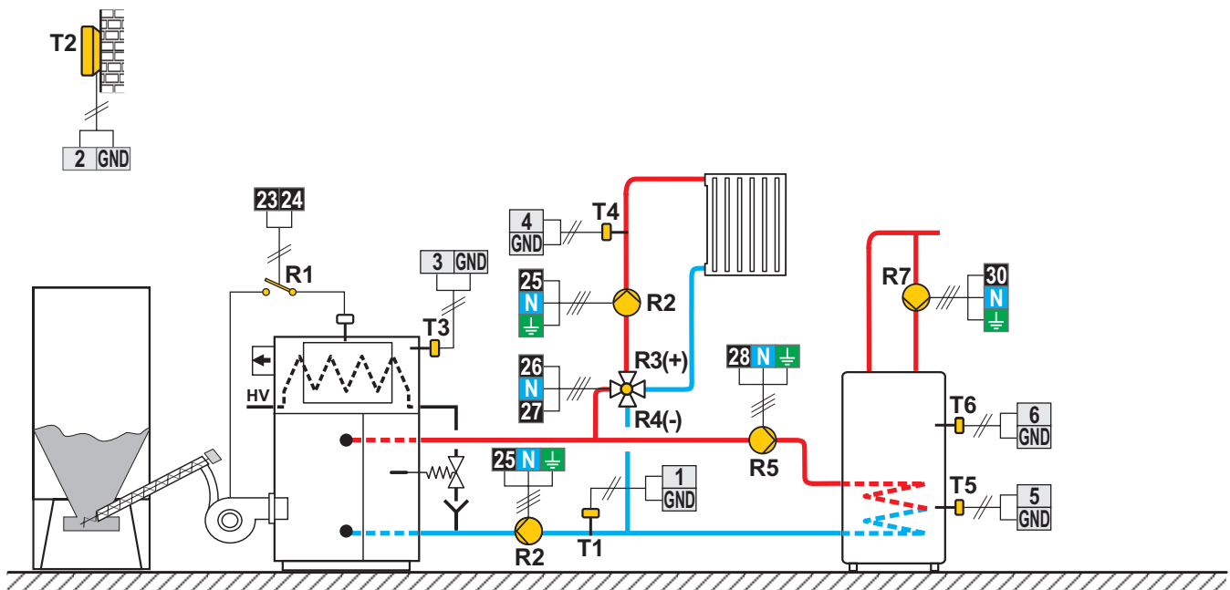
Scheme 412 (WDC20) - Chaudière à pellets, circuit mélangeur, chauffe-eau sanitaire
