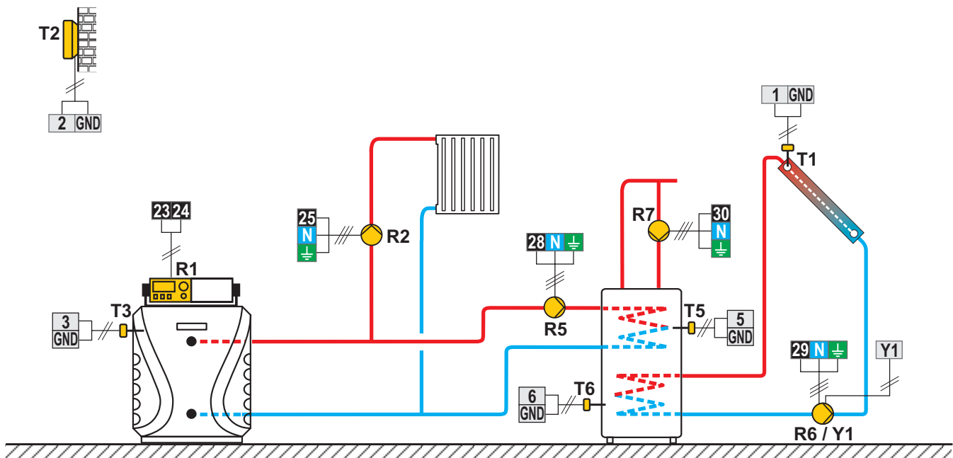
Scheme 405 (WDC10, WDC20) - Chaudière à fioul, circuit direct, chauffe-eau sanitaire, capteurs solaires
