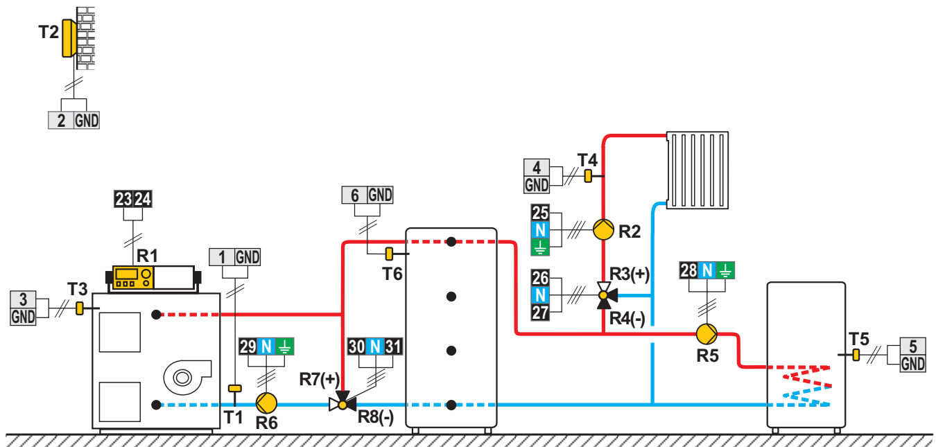
Scheme 414 (WDC20) - Chaudière combinée (combustible solide/fioul), ballon d'eau chaude, circuit mélangeur, chauffe-eau sanitaire
