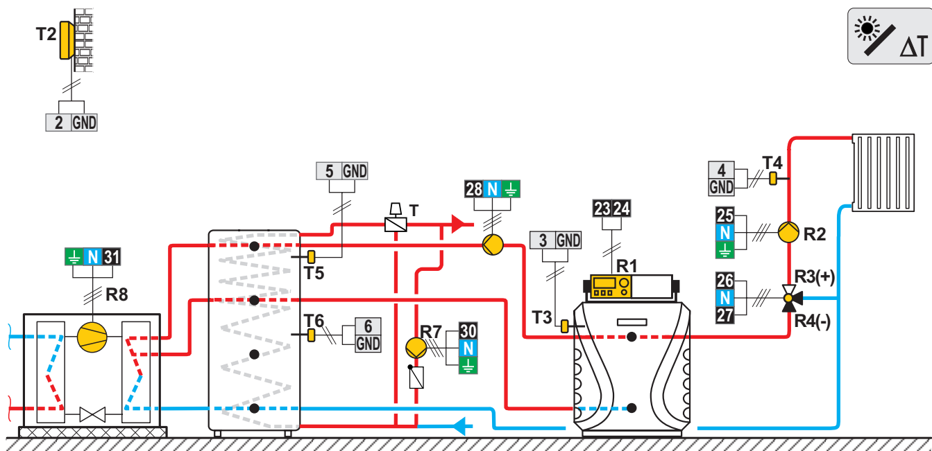
Scheme 422b (WDC20) - Pompe à chaleur, chaudière à fioul, ballon d'eau chaude avec chauffe-eau sanitaire, circuit mélangeur
