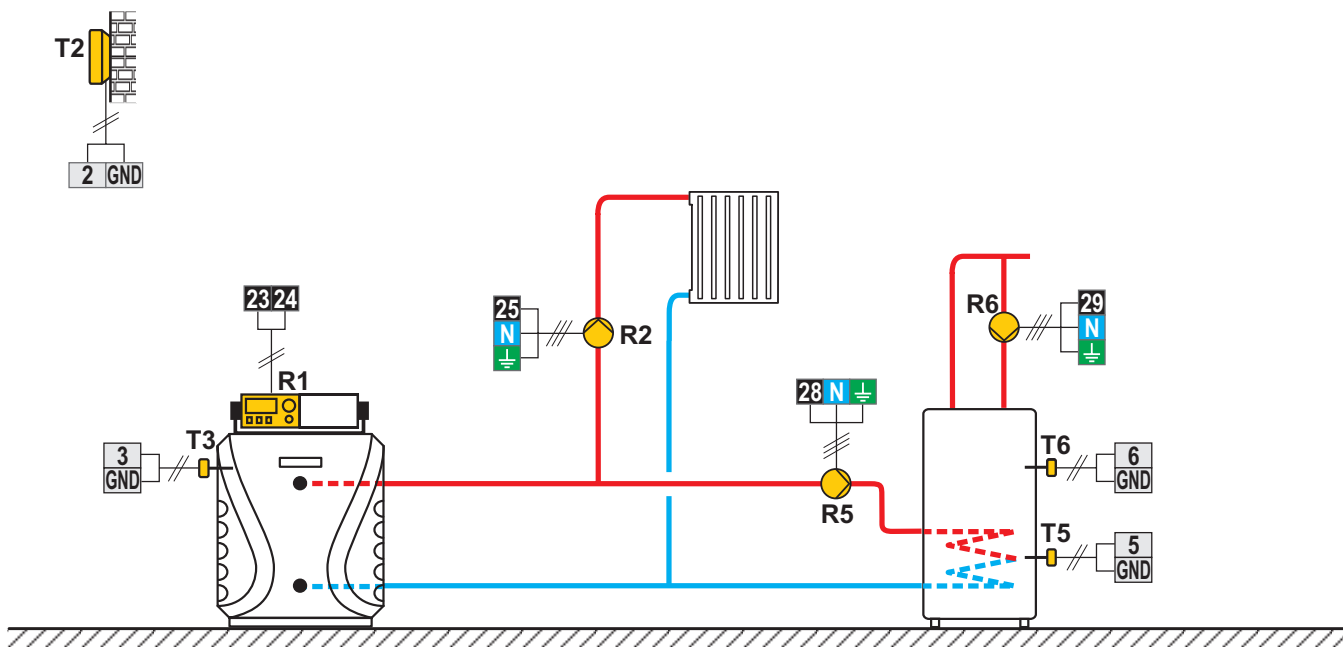
Scheme 402 (WDC10B, WDC10, WDC20) - Chaudière à fioul, circuit direct, chauffe-eau sanitaire
