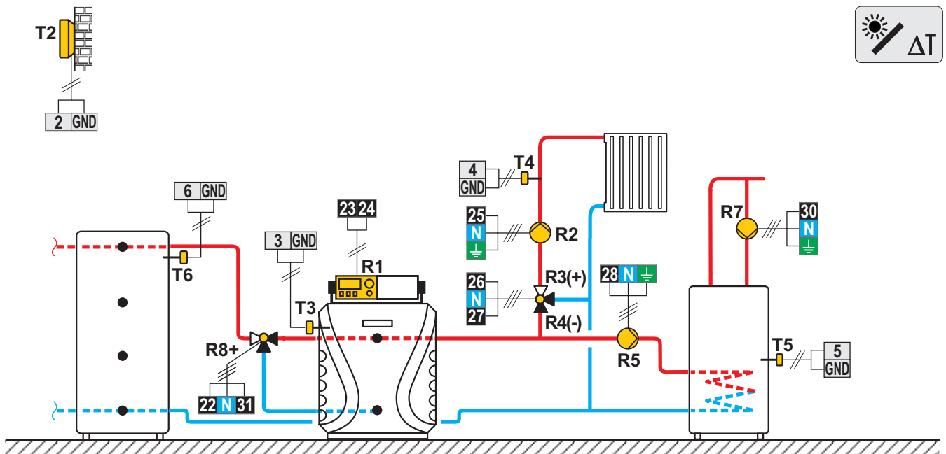
Scheme 421 (WDC20) - Chaudière à fioul, ballon d'eau chaude, circuit mélangeur, chauffe-eau sanitaire
