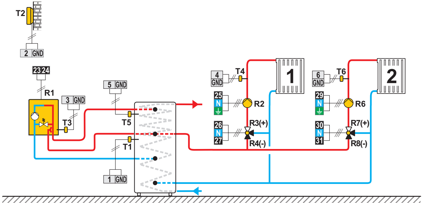
Schema 423c (WDC20) - Chaudière à gaz, ballon d'eau chaude avec chauffe-eau sanitaire int., 2x circuit mélangeur
