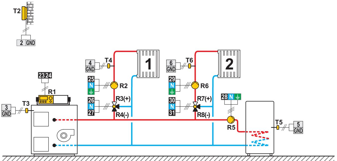
Schema 423g (WDC20) - Chaudière combinée (combustible solide/fioul), 2x circuit mélangeur, chauffe-eau sanitaire
