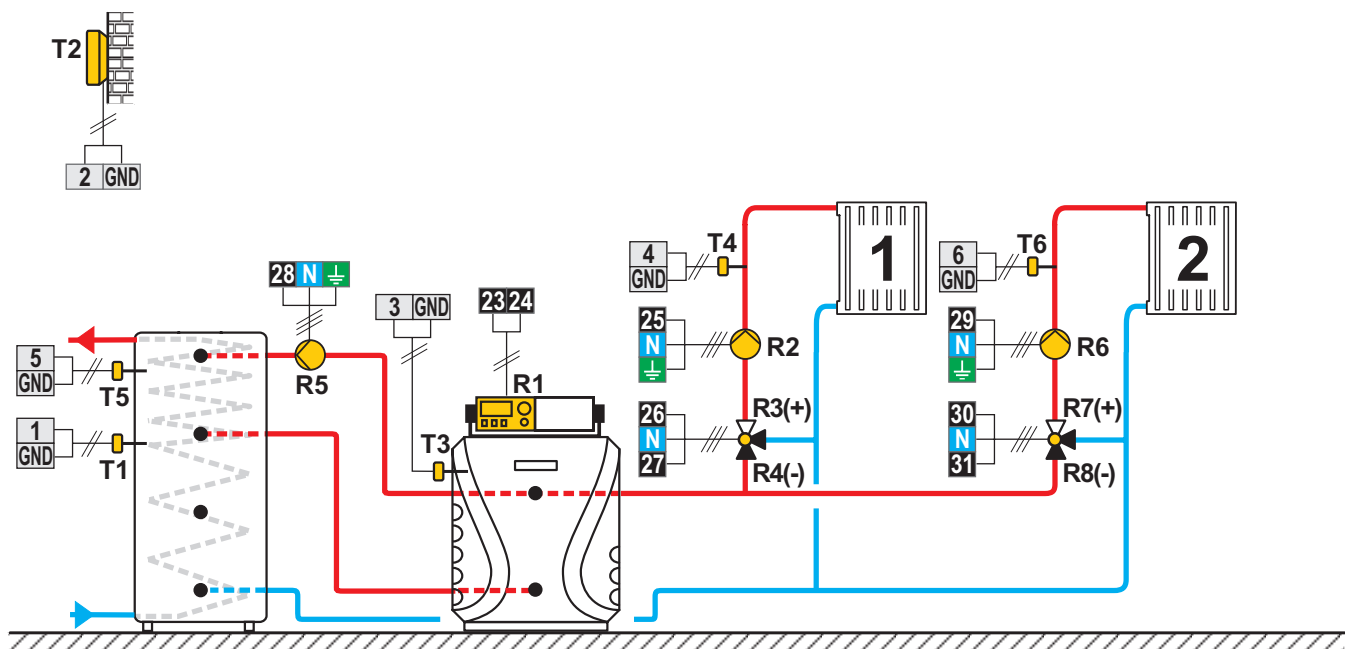
Scheme 423b (WDC20) - Chaudière à combustible liquide, ballon d'eau chaude avec chauffe-eau sanitaire int., 2x circuit mélangeur
