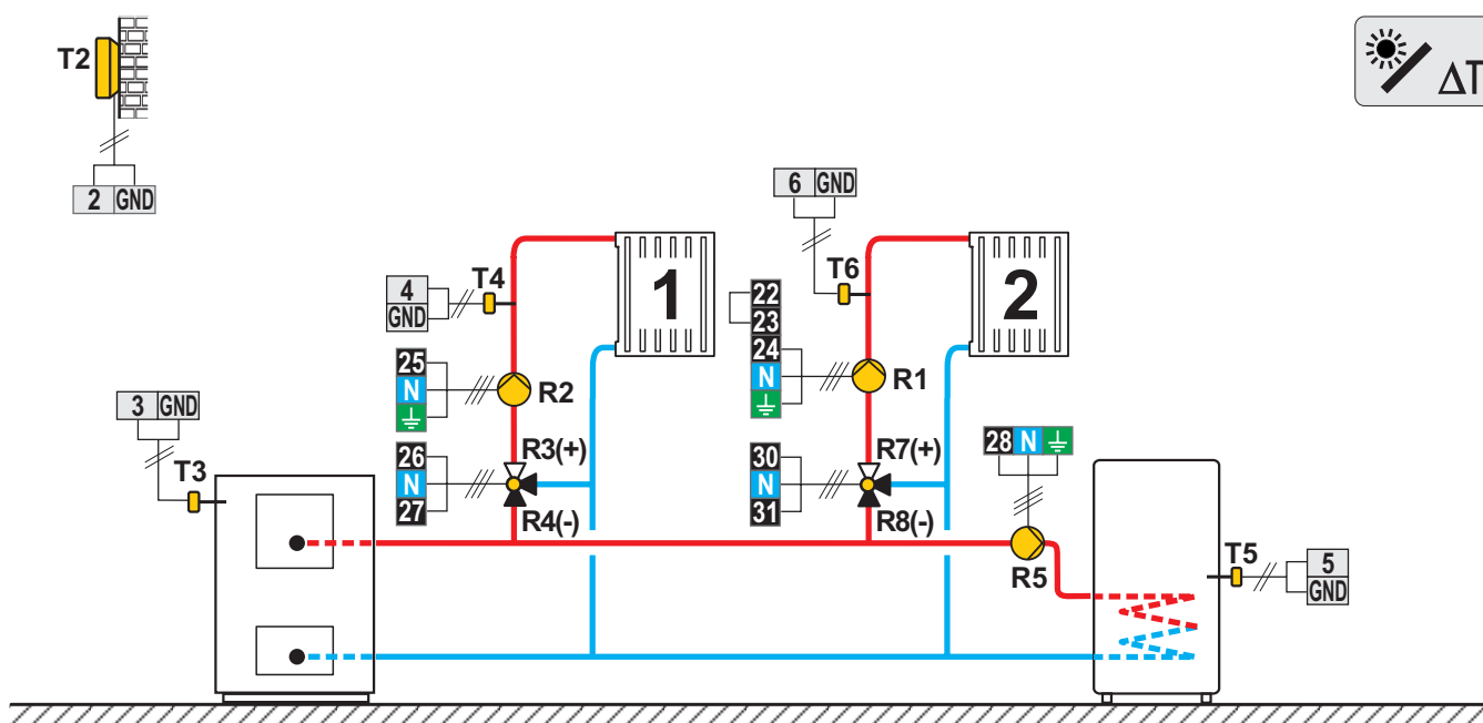
Scheme 423f (WDC20) - Chaudière à combustible solide, 2x circuit mélangeur, chauffe-eau sanitaire
