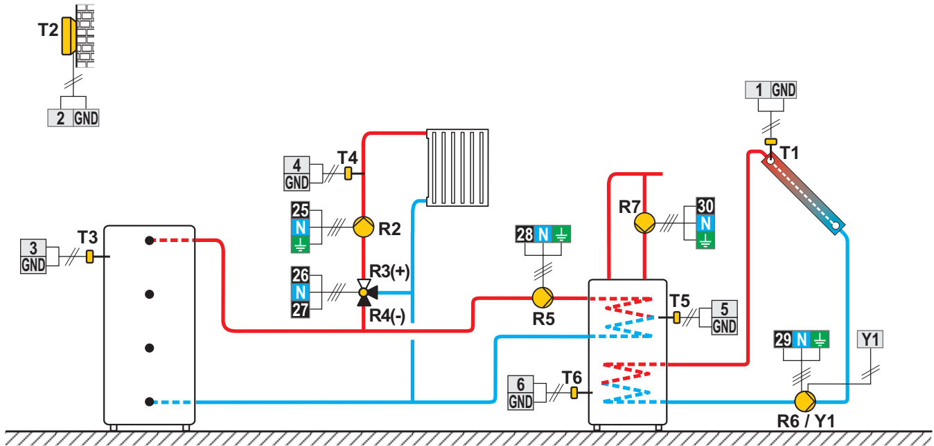
Scheme 404b (WDC10, WDC20) - Ballon d'eau chaude, circuit mélangeur, chauffe-eau sanitaire, capteurs solaires
