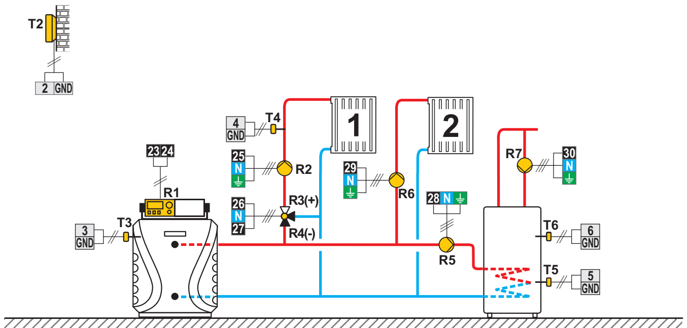
Schema 407 (WDC10, WDC20) - Chaudière à fioul, circuit direct, circuit mélangeur, chauffe-eau sanitaire
