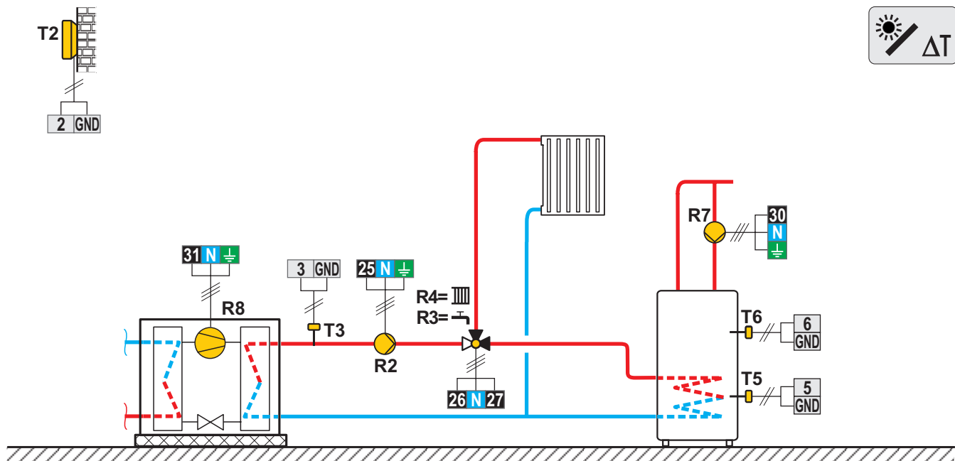
Scheme 419 (WDC20) - Pompe à chaleur, circuit direct, chauffe-eau sanitaire
