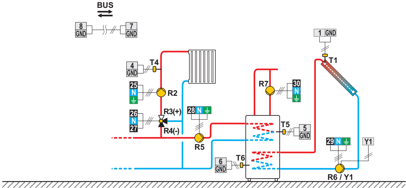
Scheme 404f (WDC10, WDC20) - Schéma d'extension - circuit mélangeur, chauffe-eau sanitaire, capteurs solaires
