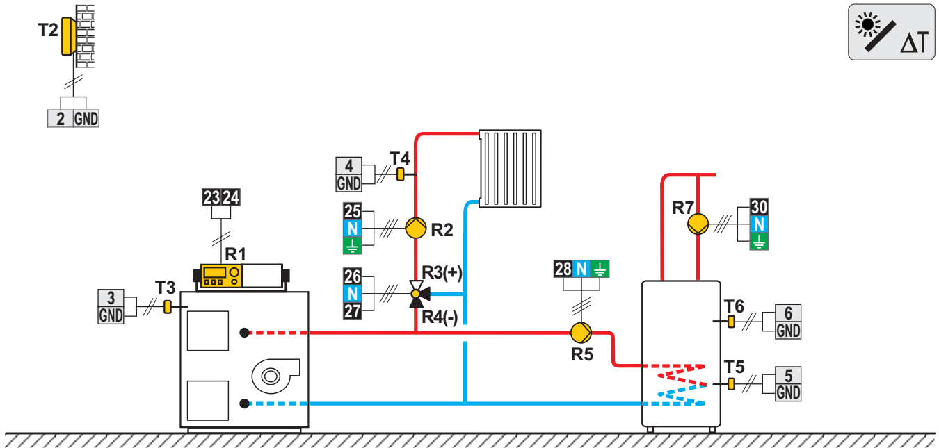
Scheme 413 (WDC20) - Chaudière combinée (combustible solide/fioul), circuit mélangeur, chauffe-eau sanitaire
