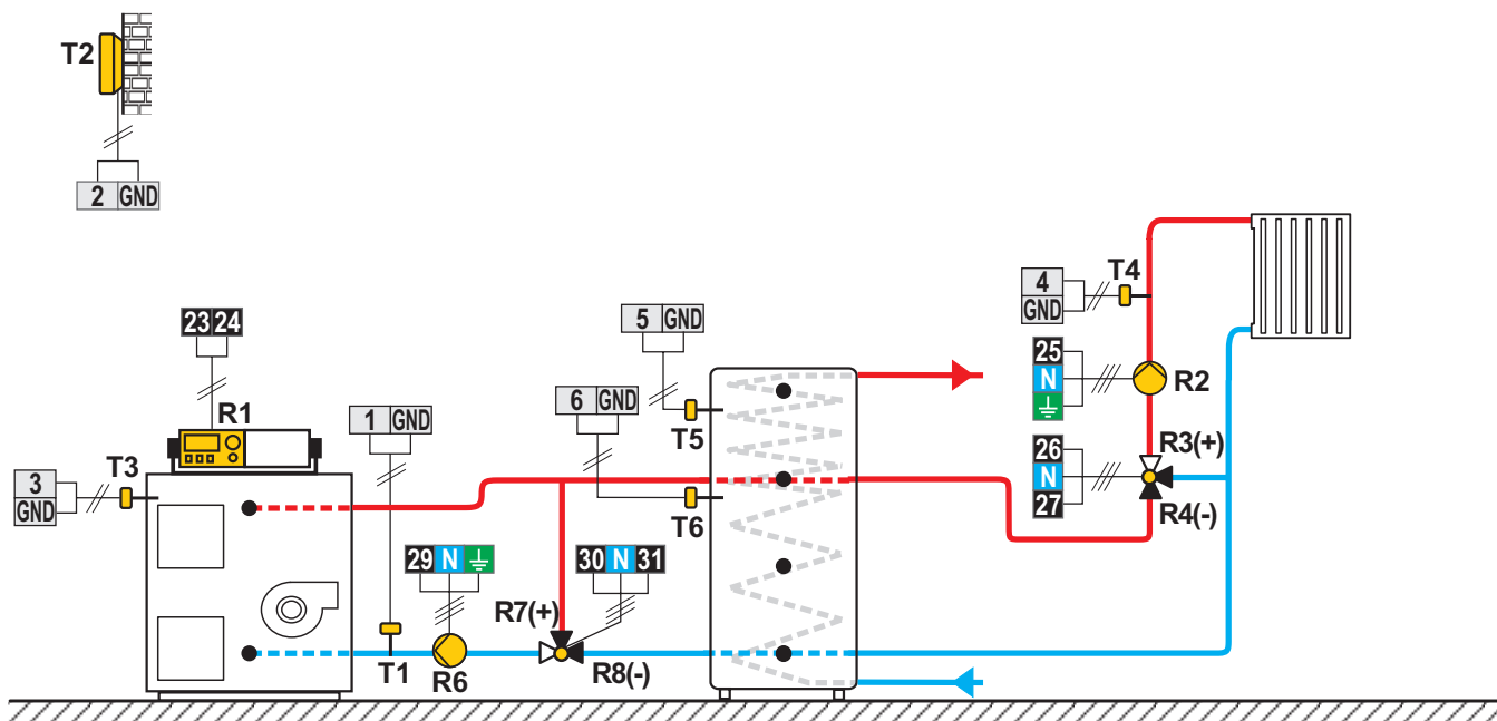
Scheme 415 (WDC20) - Chaudière combinée (combustible solide/fioul), ballon d'eau chaude avec chauffe-eau sanitaire int., circuit mélangeur
