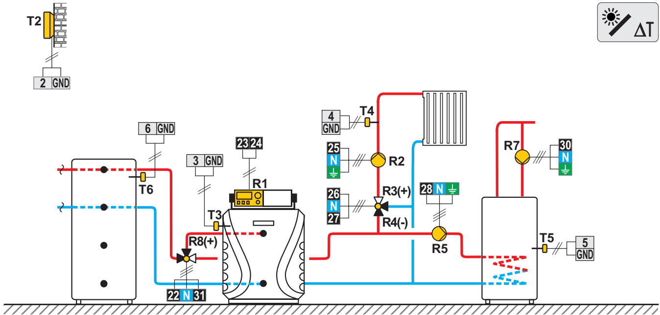
Scheme 411 (WDC20) - Ballon d'eau chaude, chaudière à fioul, circuit mélangeur, chauffe-eau sanitaire
