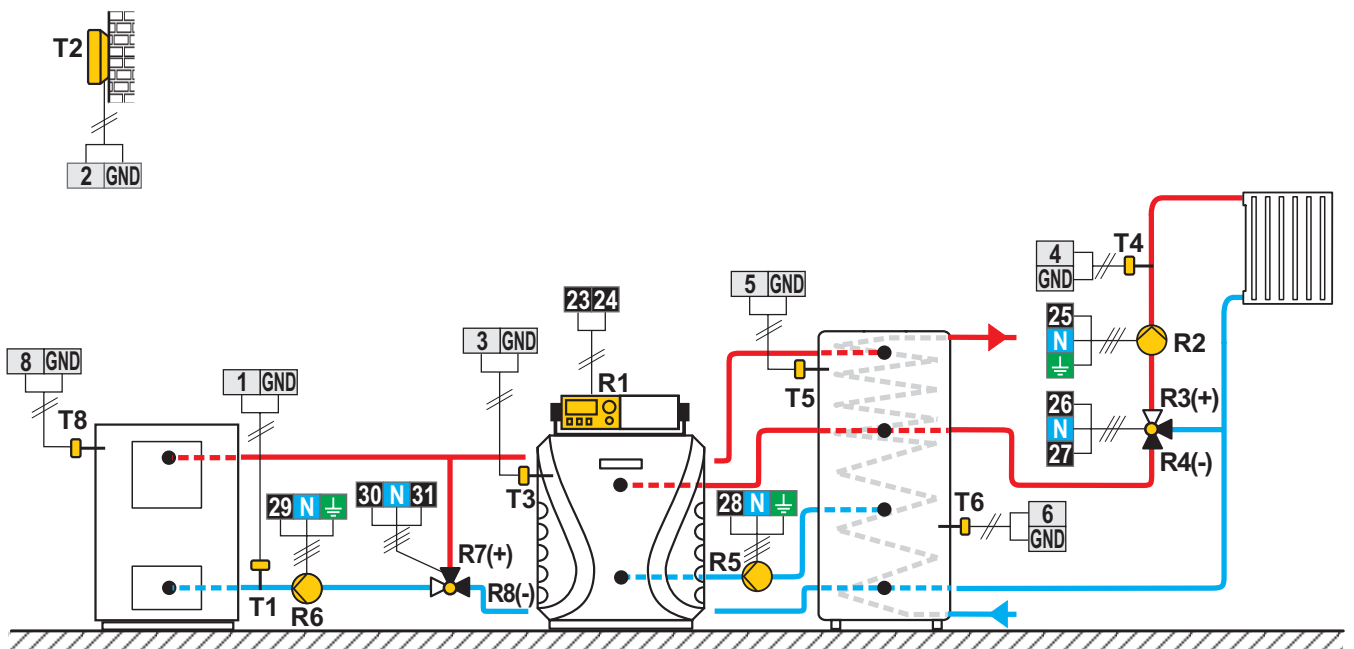
Scheme 415c (WDC20) - Chaudière à fioul, chaudière à combustible solide, ballon d'eau chaude avec chauffe-eau sanitaire intégré, circuit mélangeur
