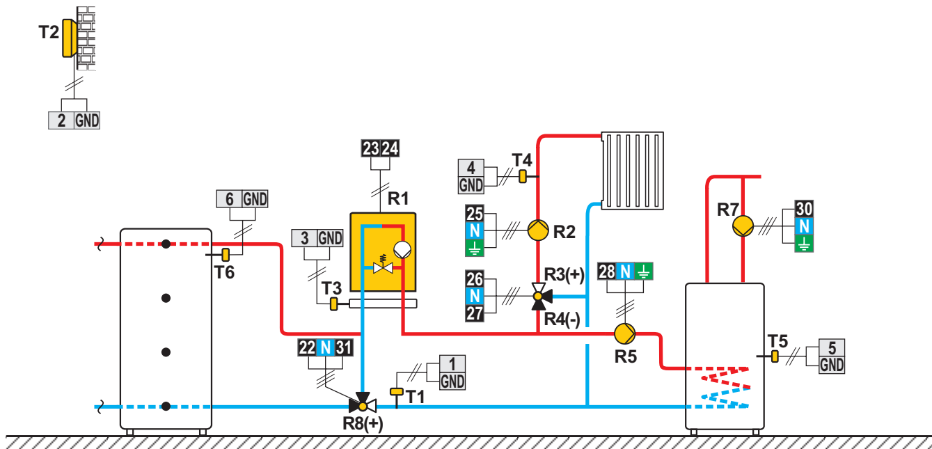
Schema 410b (WDC20) - Ballon d'eau chaude, chaudière à gaz, circuit mélangeur, chauffe-eau sanitaire
