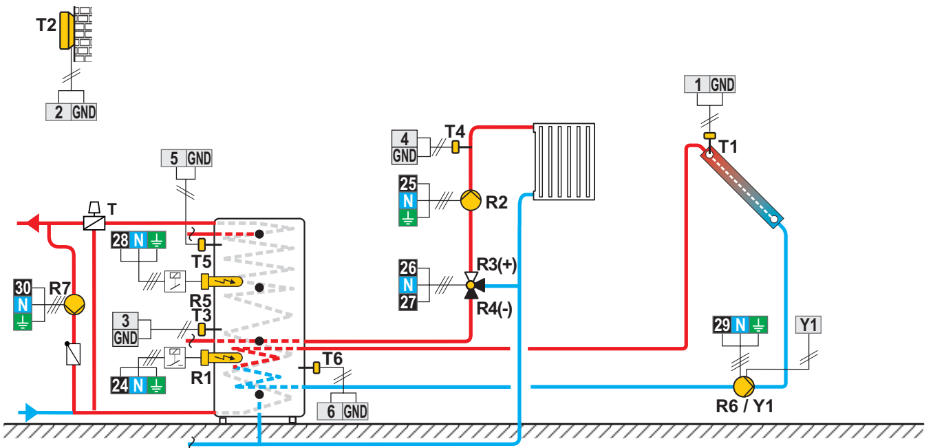
Schème 404e (WDC10, WDC20) - Ballon d'eau chaude avec chauffe-eau sanitaire intégré, circuit mélangeur, capteurs solaires
