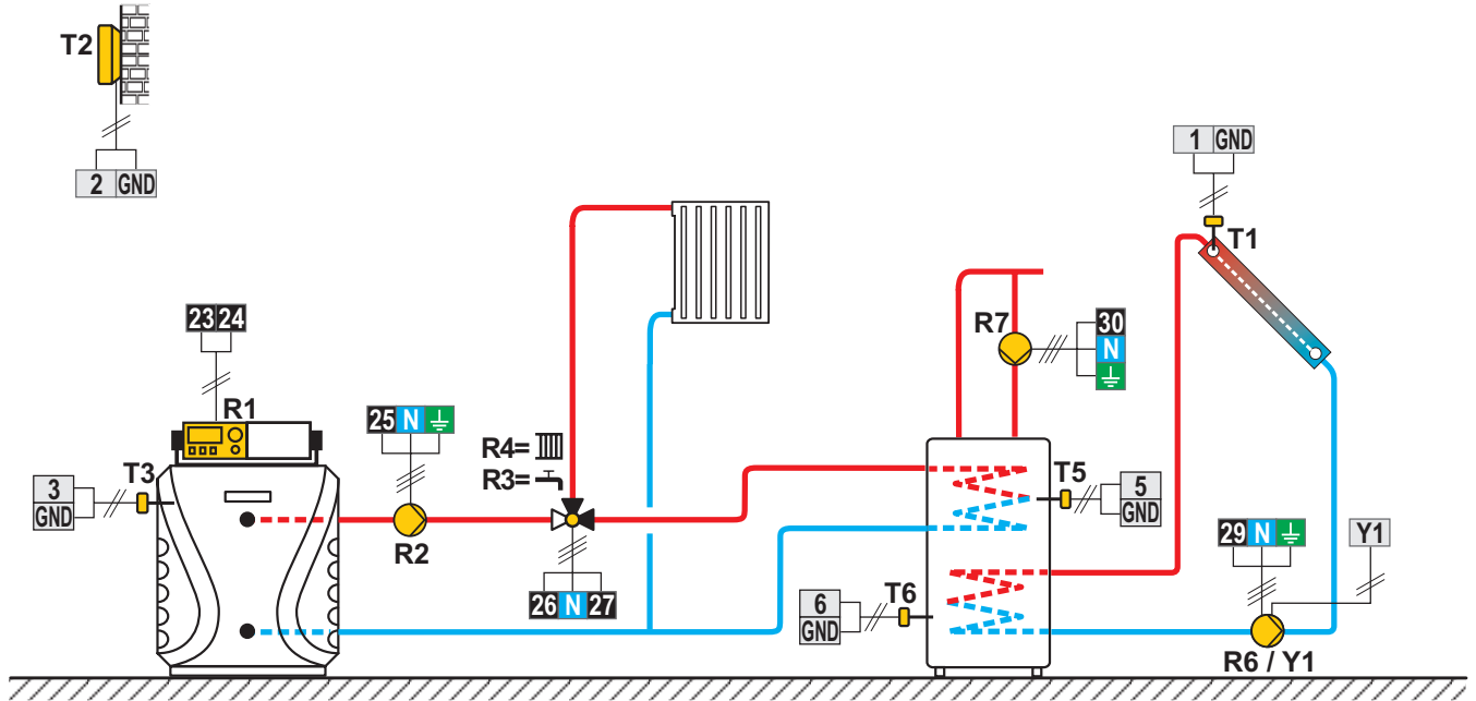
Schema 406 (WDC10, WDC20) - Chaudière à fioul, circuit direct, chauffe-eau sanitaire, capteurs solaires
