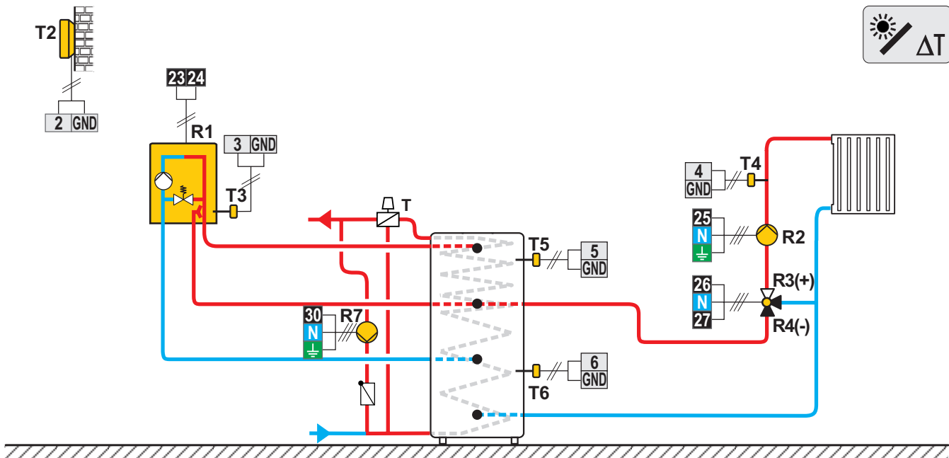
Scheme 416b (WDC20) - Chaudière à gaz, ballon d'eau chaude avec chauffe-eau sanitaire intégré, circuit mélangeur
