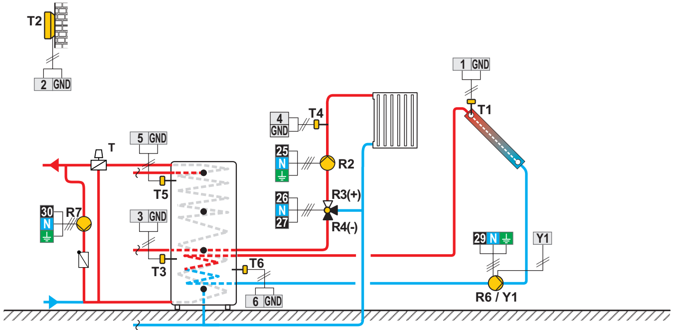
Schème 404d (WDC10, WDC20) - Ballon d'eau chaude avec chauffe-eau sanitaire intégré, circuit mélangeur, capteurs solaires
