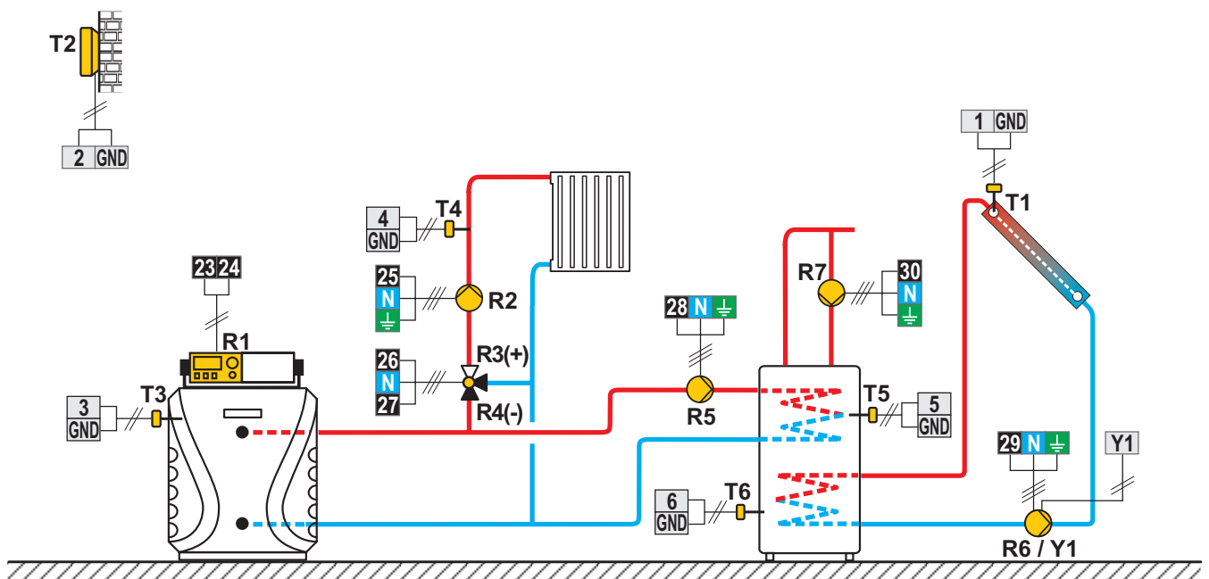
Scheme 404 (WDC10, WDC20) - Chaudière à fioul, circuit mélangeur, chauffe-eau sanitaire, capteurs solaires
