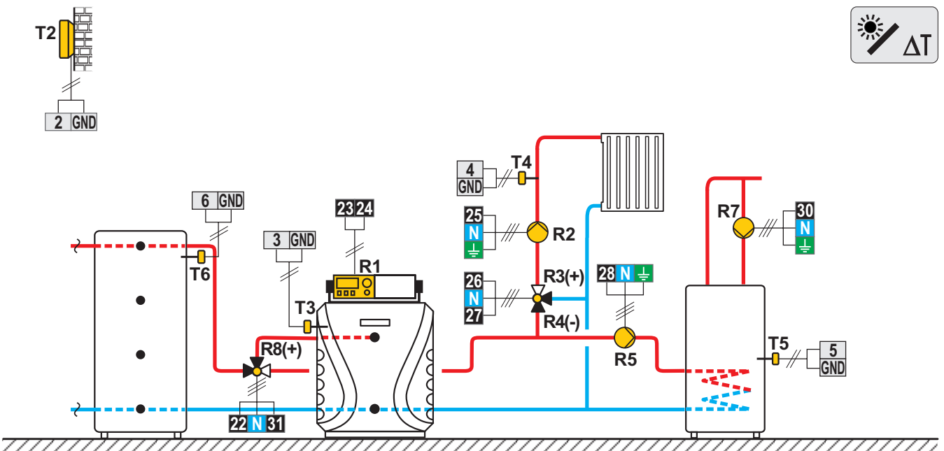
Scheme 409 (WDC20) - Ballon d'eau chaude, chaudière à fioul, circuit mélangeur, chauffe-eau sanitaire
