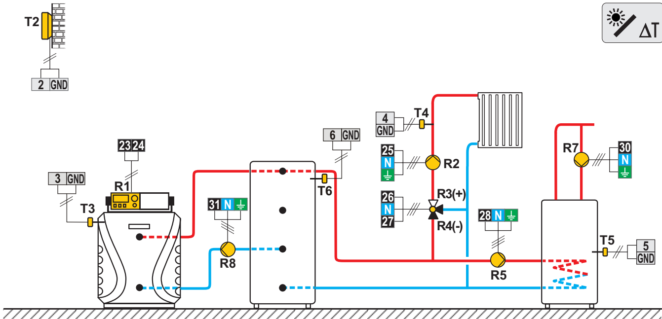
Scheme 416 (WDC20) - Chaudière à fioul, ballon d'eau chaude, circuit mélangeur, chauffe-eau sanitaire
