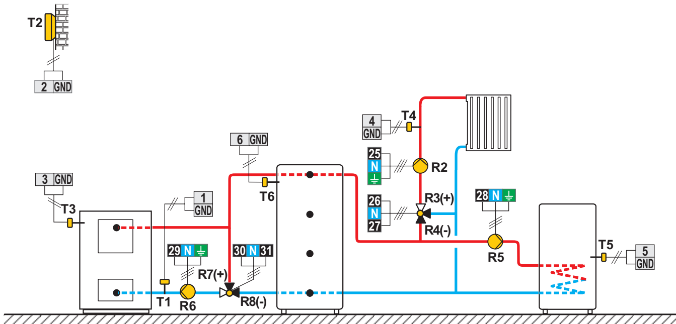
Scheme 414b (WDC20) - Chaudière à combustible solide, ballon d'eau chaude, circuit mélangeur, chauffe-eau sanitaire
