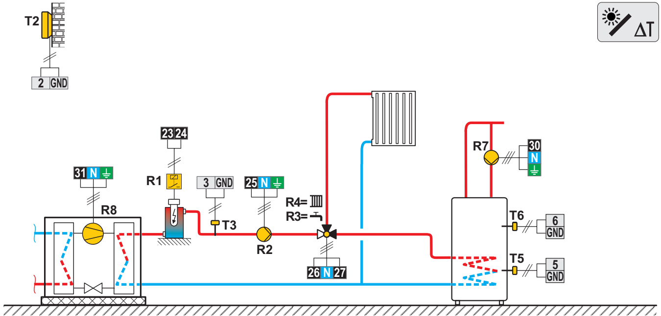
Scheme 420 (WDC20) - Pompe à chaleur, chauffage électrique d'appoint, circuit direct, chauffe-eau sanitaire
