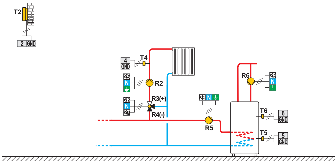
Scheme 401d (WDC10B, WDC10, WDC20) - Système sans chaudière - circuit mélangeur, chauffe-eau sanitaire
