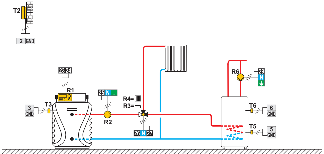
Scheme 403 (WDC10B, WDC10, WDC20) - Chaudière à fioul, circuit direct, chauffe-eau sanitaire
