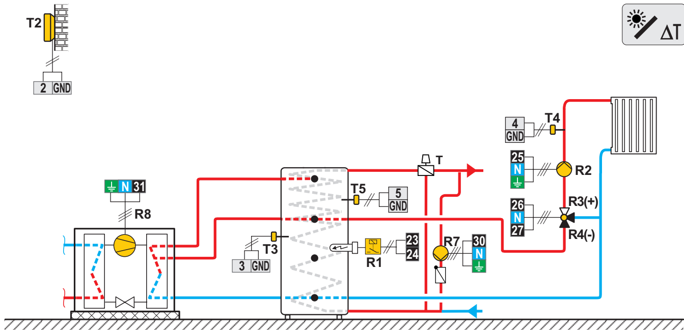
Scheme 422 (WDC20) - Pompe à chaleur, ballon d'eau chaude avec chauffe-eau sanitaire int., circuit mélangeur
