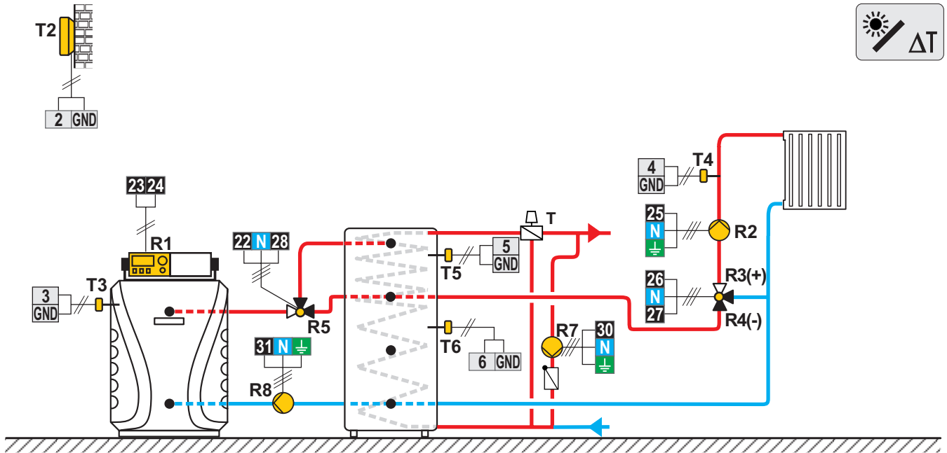
Scheme 416c (WDC20) - Chaudière à fioul, ballon d'eau chaude avec chauffe-eau sanitaire intégré, circuit mélangeur
