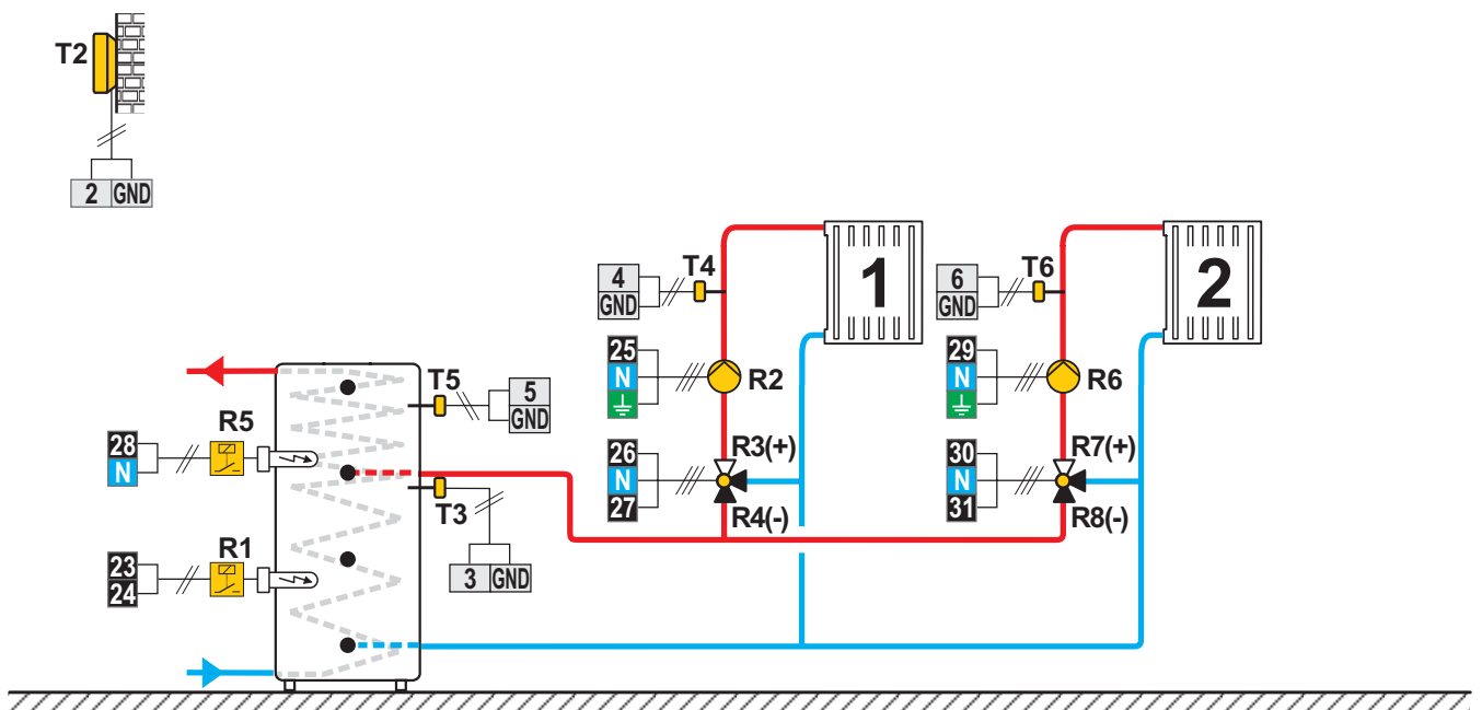
Schema 423d (WDC20) - Schéma d'extension - ballon d'eau chaude avec chauffe-eau sanitaire int., 2x circuit mélangeur
