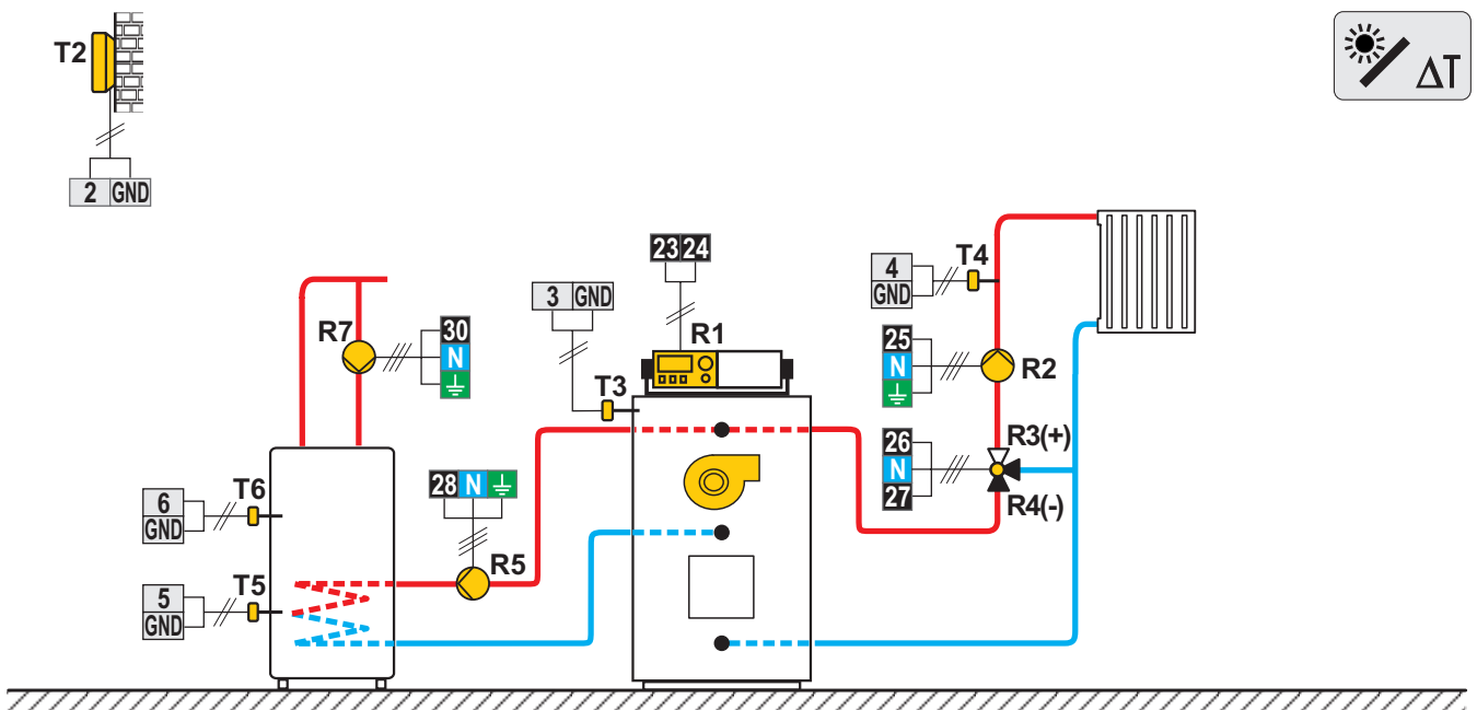
Scheme 417 (WDC20) - Chaudière combinée (combustible solide/fioul), circuit mélangeur, chauffe-eau sanitaire
