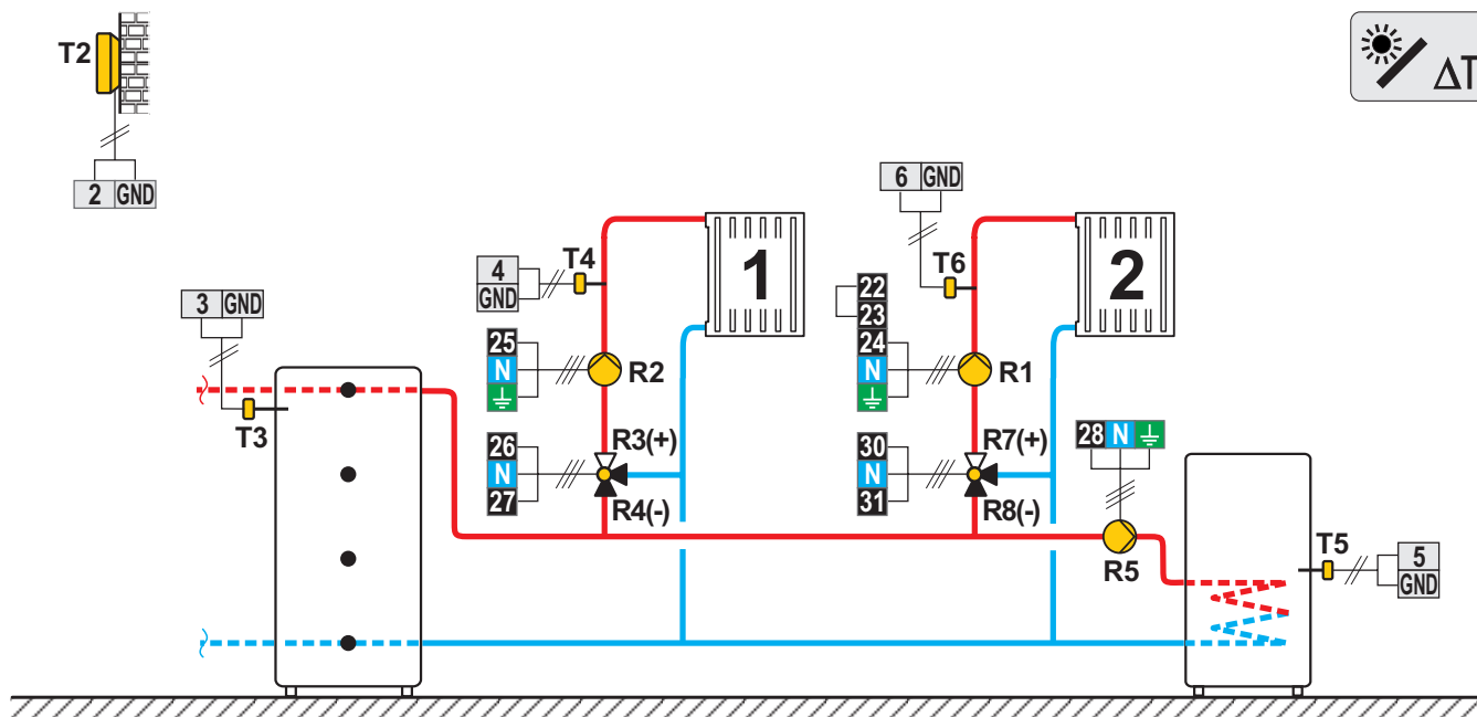
Scheme 423e (WDC20) - Ballon d'eau chaude, 2x circuit mélangeur, chauffe-eau sanitaire
