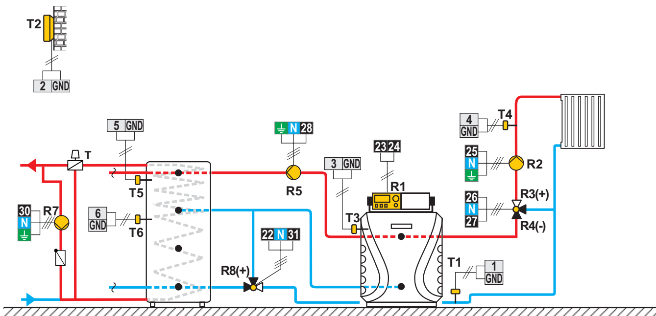
Schema 410c (WDC20) - Ballon d'eau chaude avec chauffe-eau sanitaire int., chaudière à fioul, circuit mélangeur
