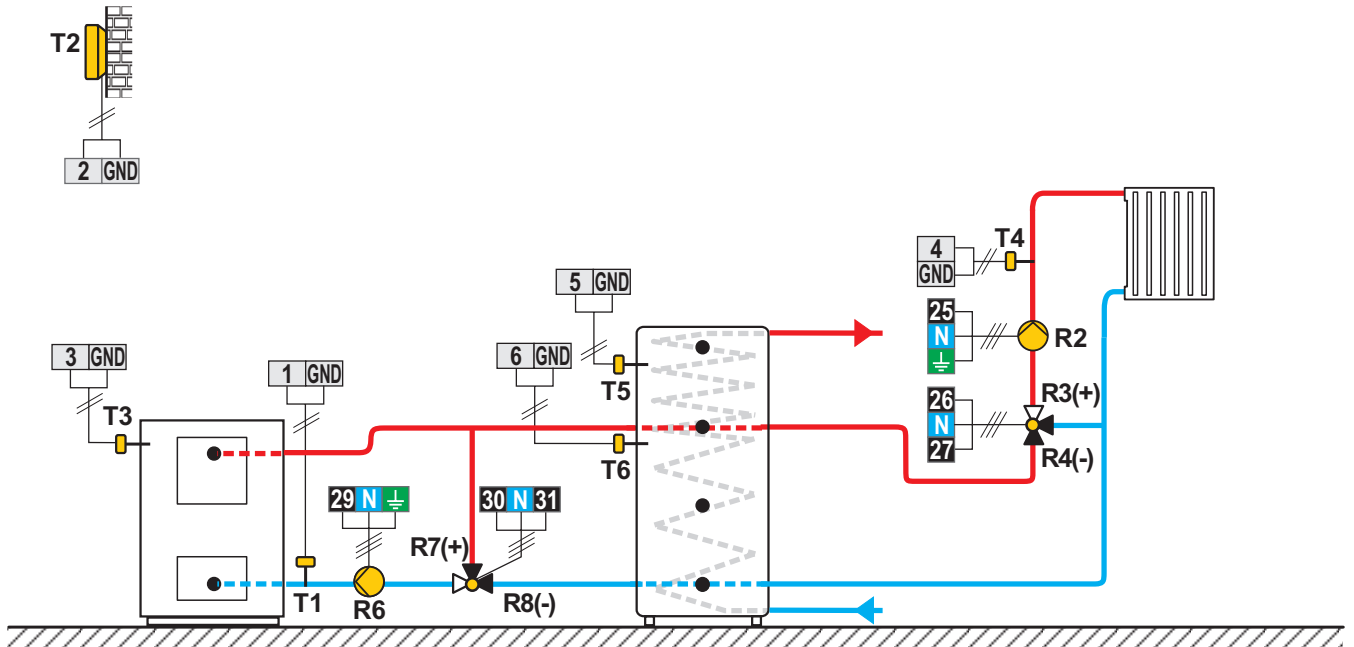
Scheme 415b (WDC20) - Chaudière à combustible solide, ballon d'eau chaude, circuit mélangeur, chauffe-eau sanitaire
