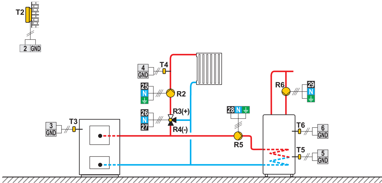
Scheme 401c (WDC10B, WDC10, WDC20) - Chaudière à fioul, circuit mélangeur, chauffe-eau sanitaire
