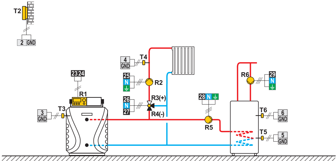
Scheme 401 (WDC10B, WDC10, WDC20) - Chaudière à fioul, circuit mélangeur, chauffe-eau sanitaire
