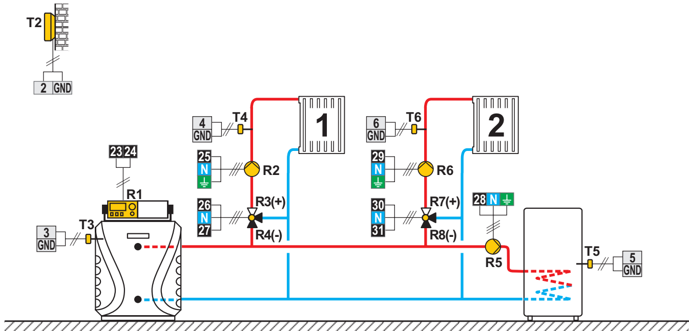
Scheme 423 (WDC20) - Chaudière à fioul, 2x circuit mélangeur, chauffe-eau sanitaire
